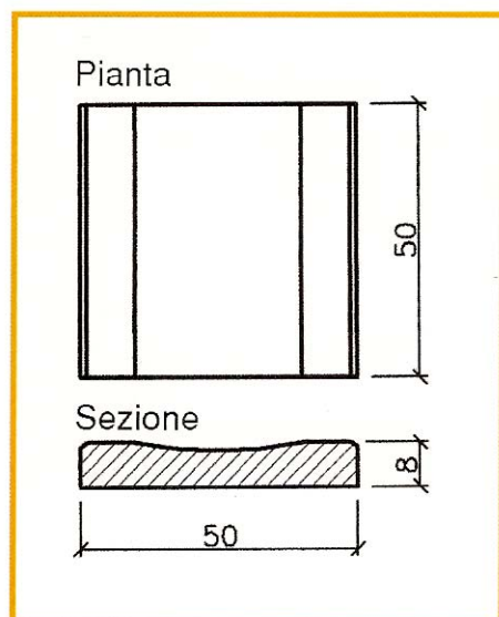
CUNETTA TIPO CREMA
