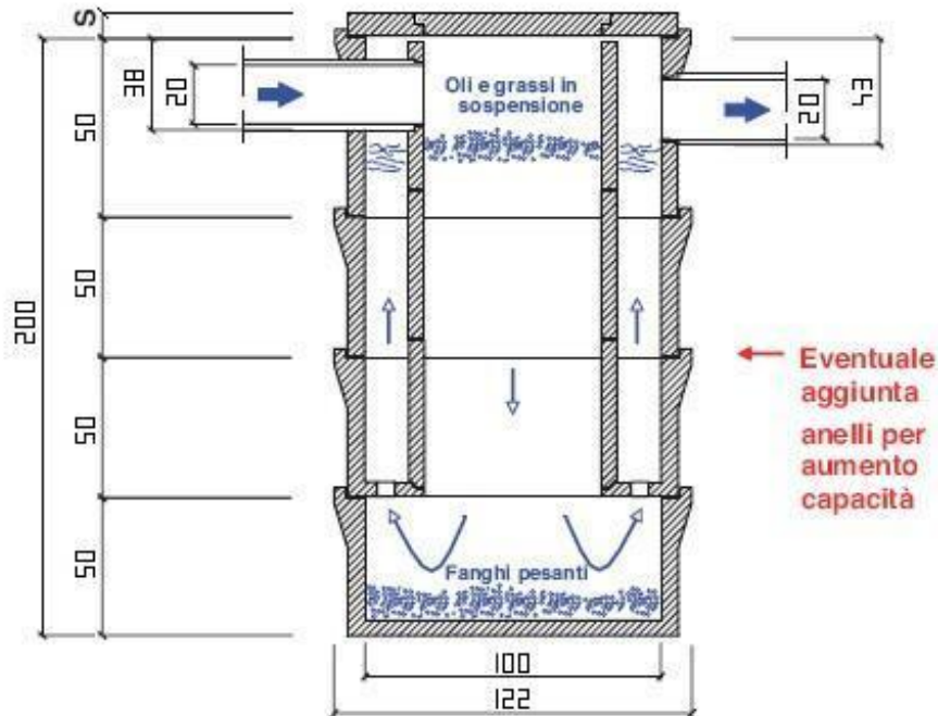
Sezione
