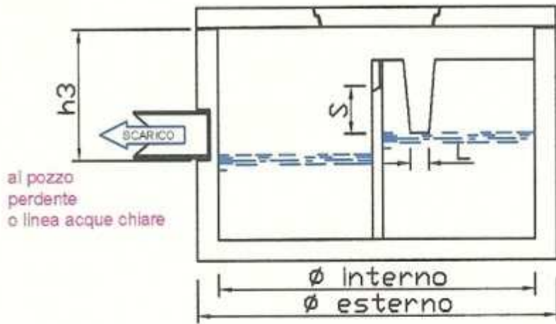
Sezione B-B
