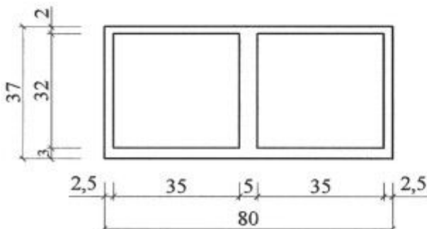
Sezione trasversale
