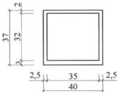
Sezione trasversale
