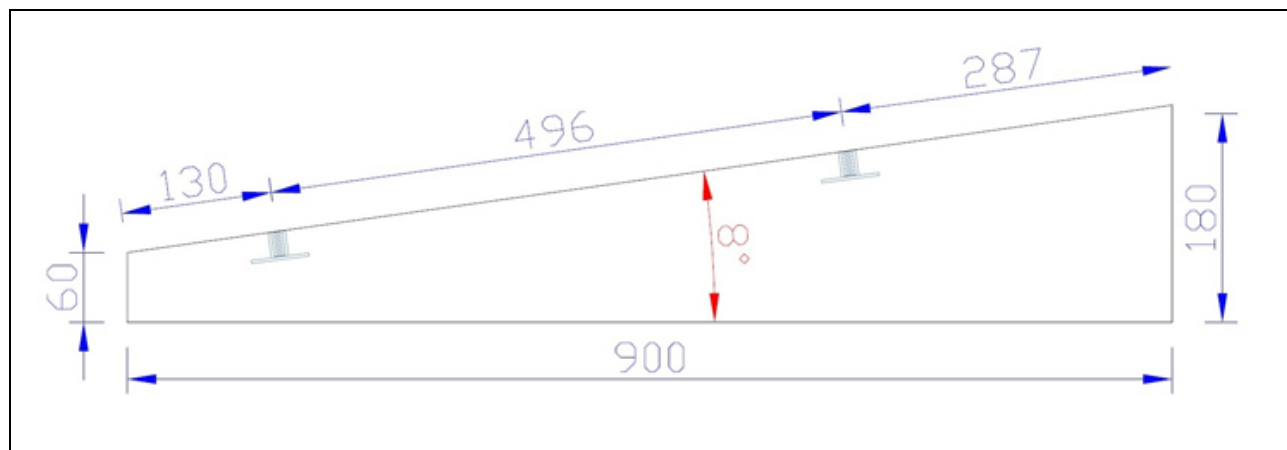
ZAVORRA CLS CM 90 incl. 8° peso kg 47
