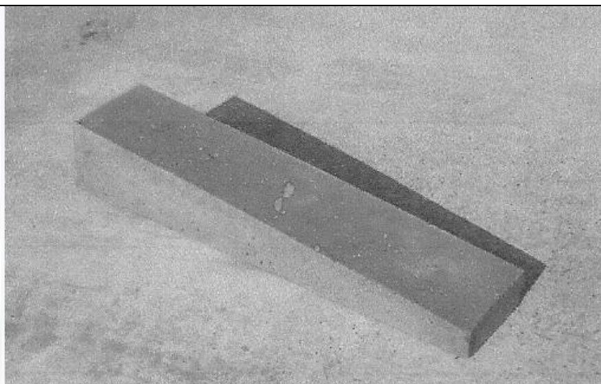
ZAVORRA CLS CM 90 incl. 8° peso kg 47
